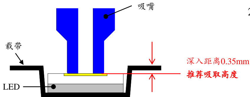
图5. 吸取高度（日亚推荐）
