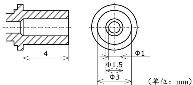
图2. 吸嘴形状例 (日亚推荐)
