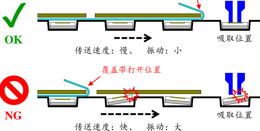
图4. 覆盖带打开位置
